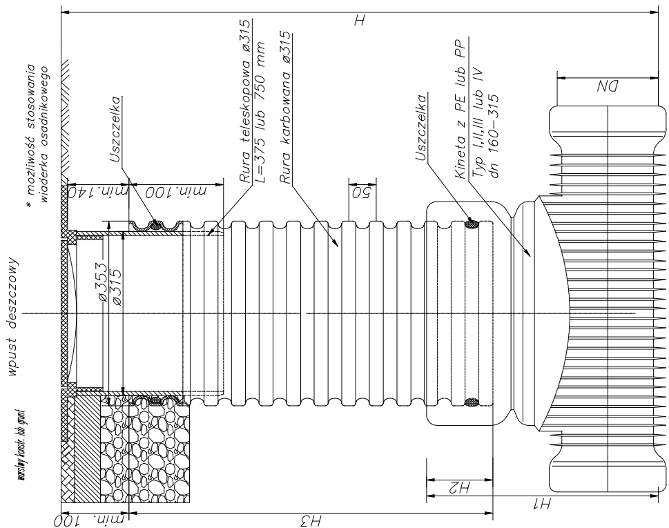
Studzienka inspekcyjna \varnothing 315
